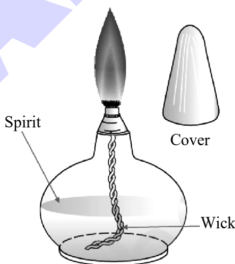
Fig. 1.14 : The spirit lamp
